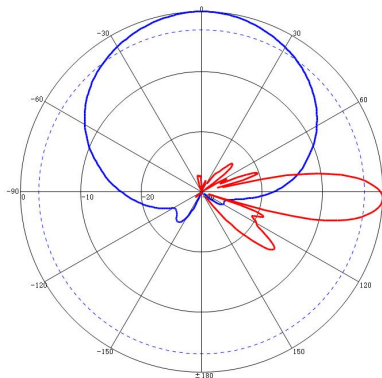
1710-2490MHz: ±45° Pol.
