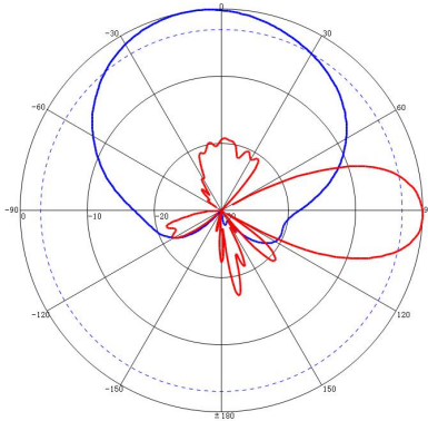
698-960MHz: ±45° Pol.
