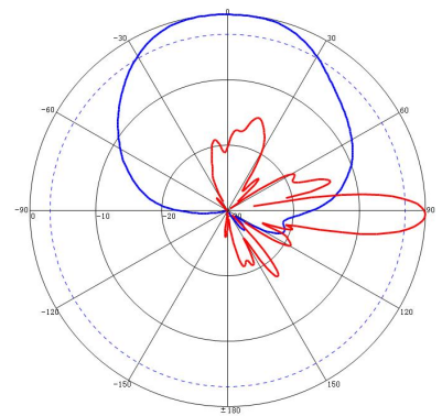
2490-2690MHz: ±45° Pol.
